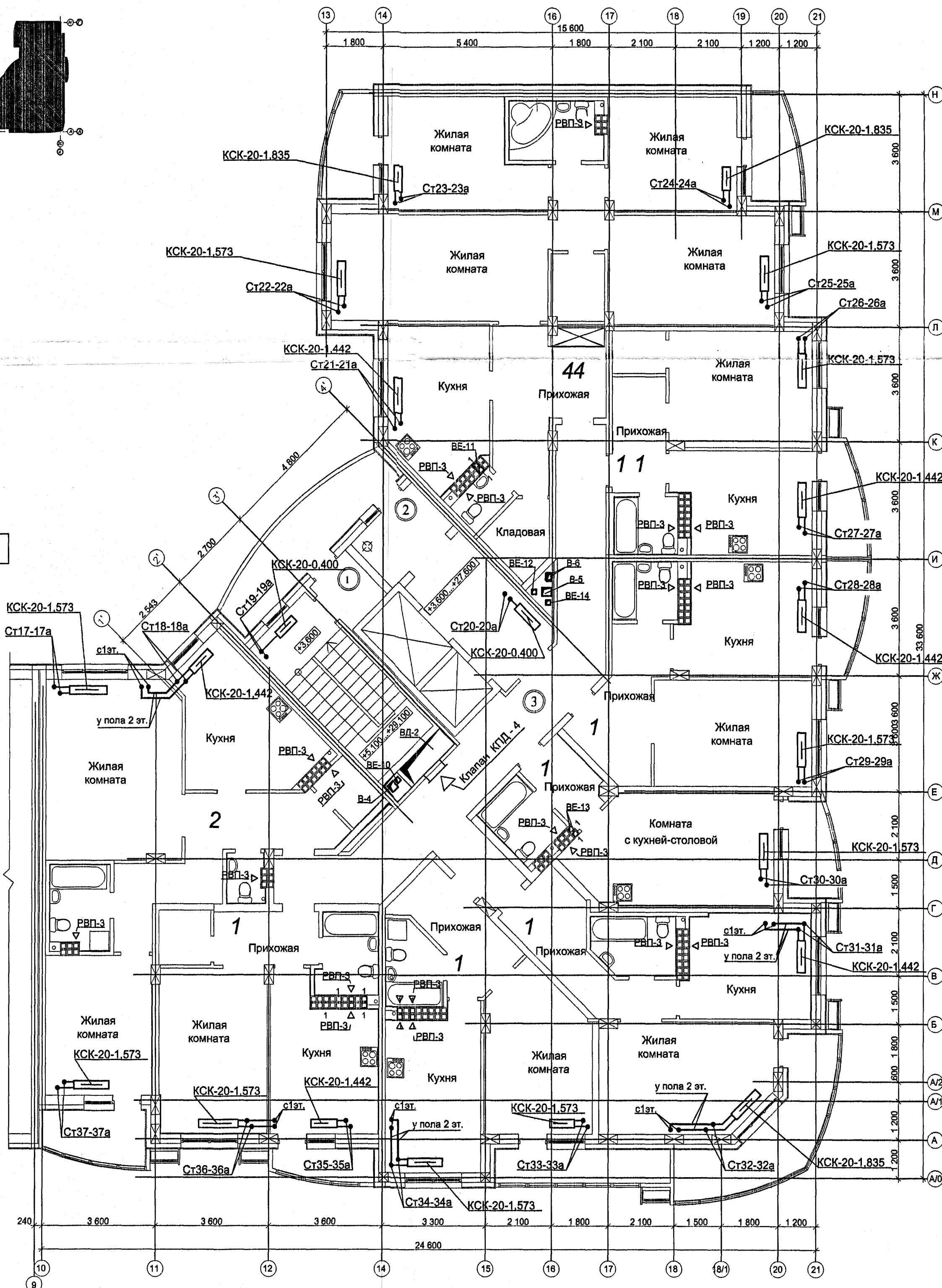
План 2-10 этажа.
